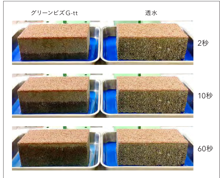
着色した水を張ったバットにグリーンビズG-tt (左) と透水製品 (右) を置いたもの。グリーンビズG-ttは配置直後に吸い上げを始め、60秒後には表層近くまで浸透しています。
