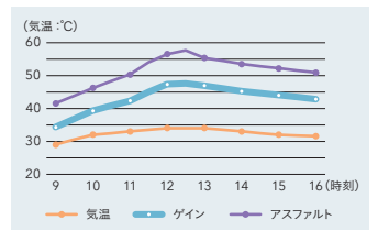
舗装面の温度履歴の比較 (湿潤) 一例
